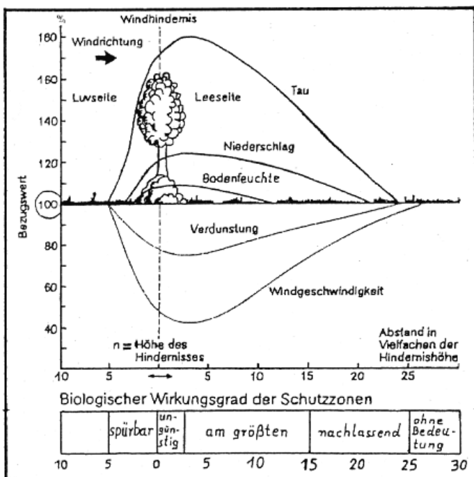
Abb. 3: Die Graphik verdeutlicht zusammengefasst die positiven Wirkungen einer Feldhecke auf die angrenzenden Ackerflächen. Taubildung, Niederschläge und Bodenfeuchtigkeit werden (vor allem auf der Lee-seite) erhöht, während sich Verdunstung und Windgeschwindigkeit verringern. (Aus Tetra nach Nägeli (1943) und Kreuz (1973), verändert).
