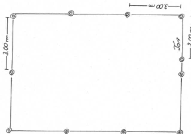
In der Schemazeichnung ist dargestellt, wie der Wildschutzzaun aufgebaut sein kann, welche Abstände sinnvoll sind.
